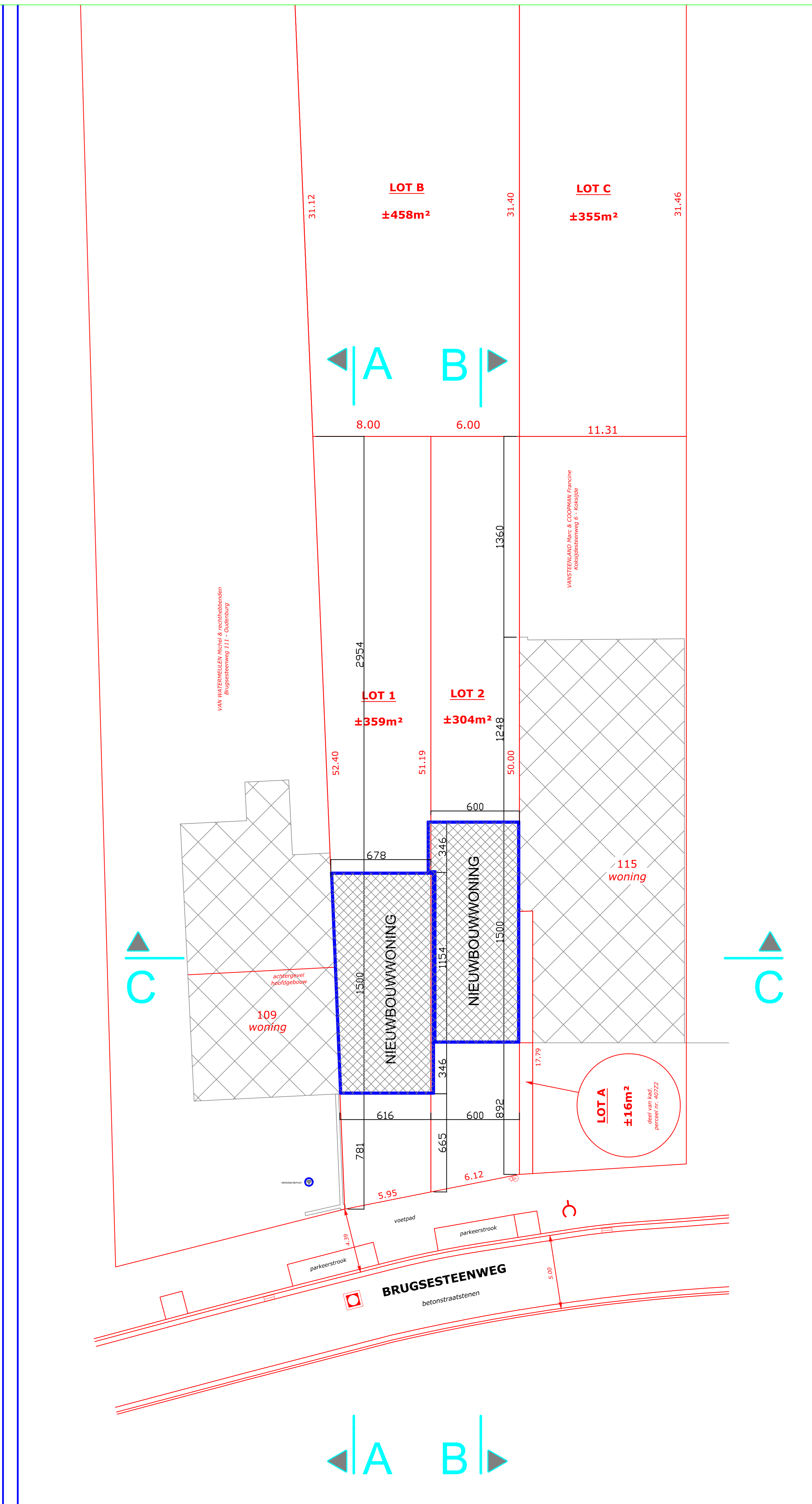
NIEUWE TOESTAND 1/200
