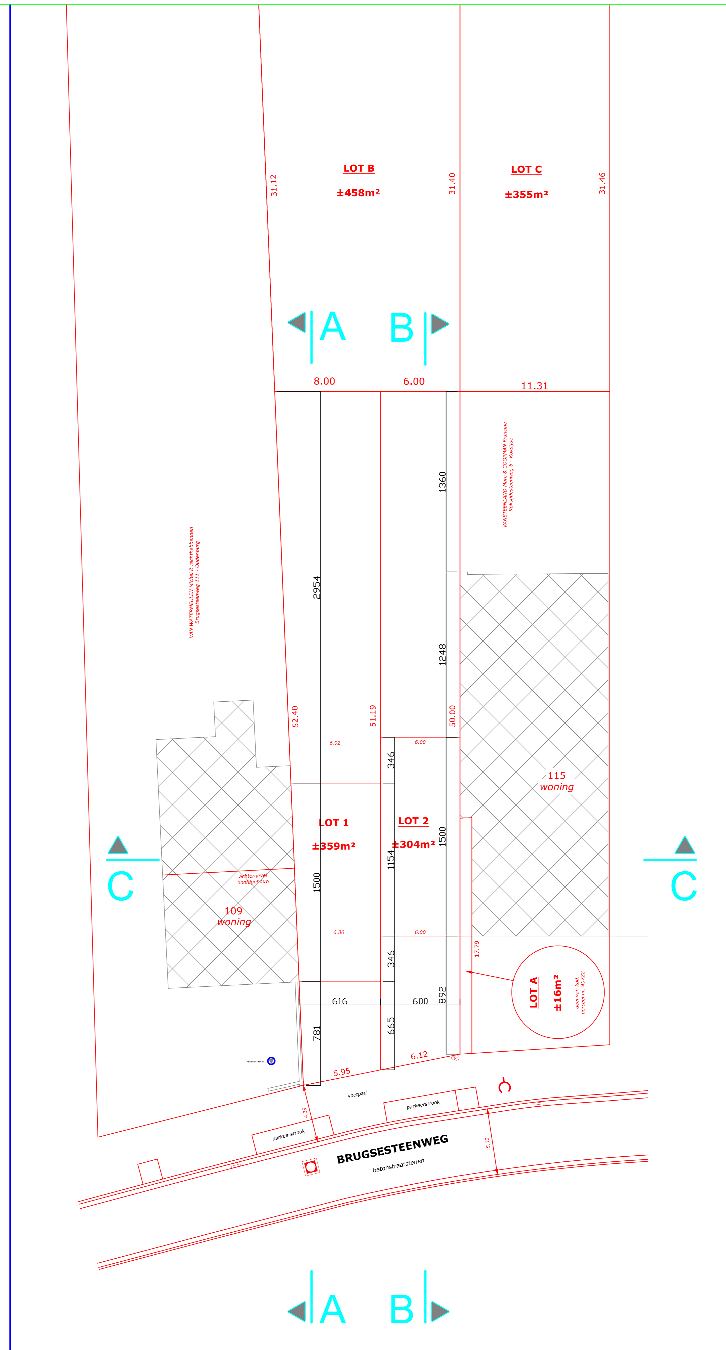
TOESTAND NA AFBRAAK 1/200
